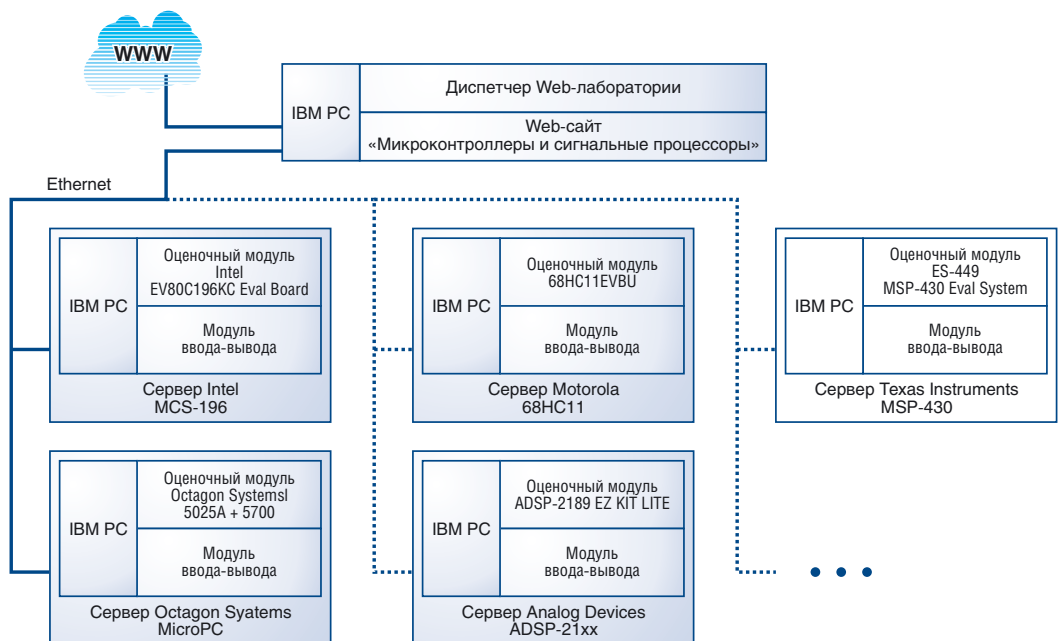
Рис. 6. Перспективная Web-лаборатория (действующие компоненты Web-лаборатории выделены синим цветом)
