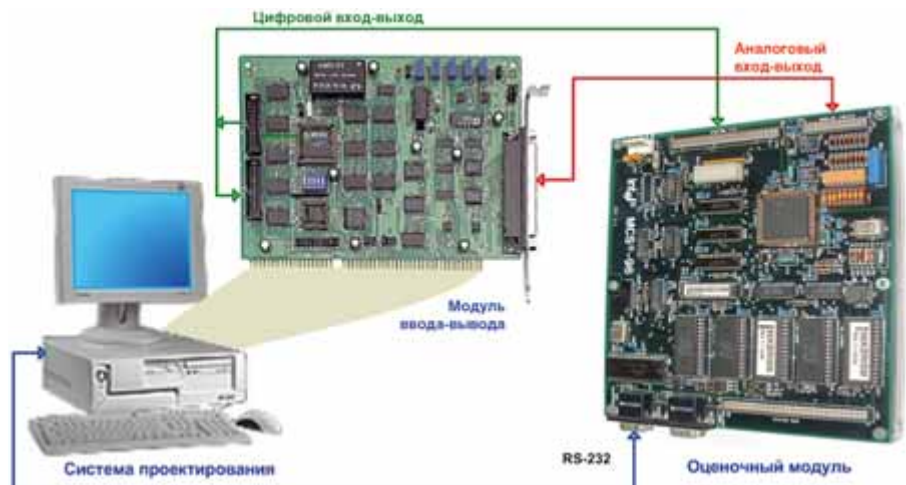
Рис. 2. Виртуальный лабораторный стенд
